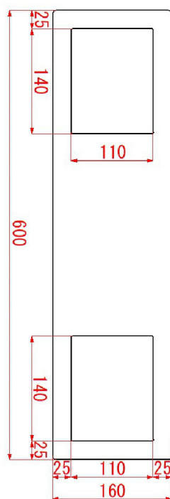
敷板寸法図面 (mm)
